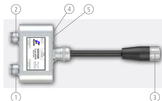
(1) Avvitatore KDS #1 (2) Avvitatore KDS #2 (3) Unità di controllo KDU (4) Pin GND (5) Pin IN
